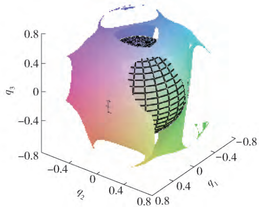
图3 机构位于给定位置的无奇异姿态球
