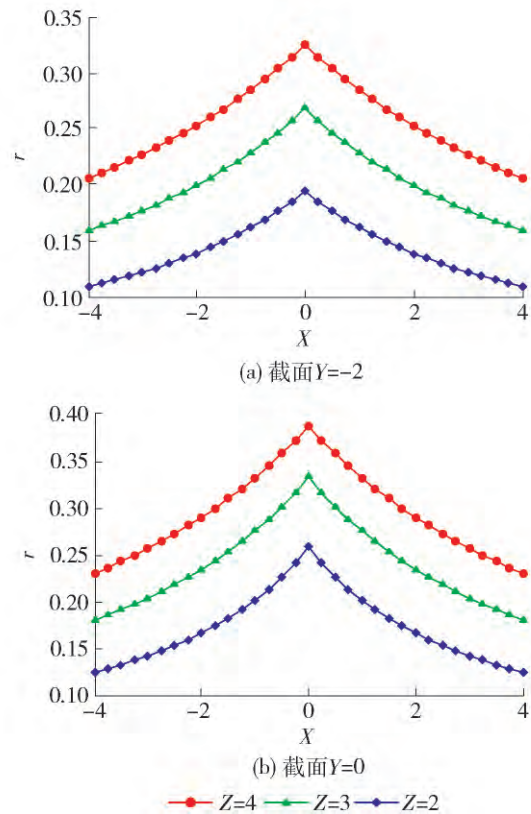
图 9 Y-截面上 r 随位置参数 X 变化 Fig. 9 r versus position parameter X in Y -sections
